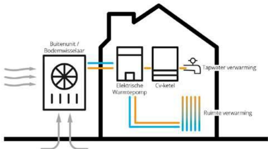
Figuur 6.3 Hybride lucht- of bodemwarmtepomp
